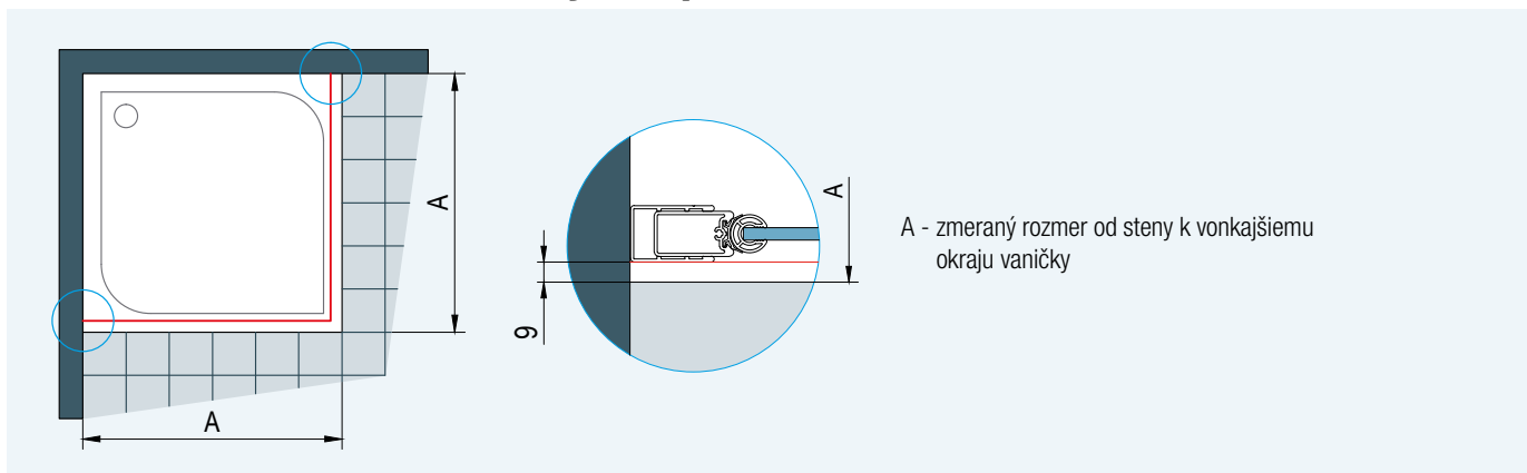
Obr. 1 Pri montáži na vaničku je odsadenie u všetkých štandardných rozmerov 9 mm.
