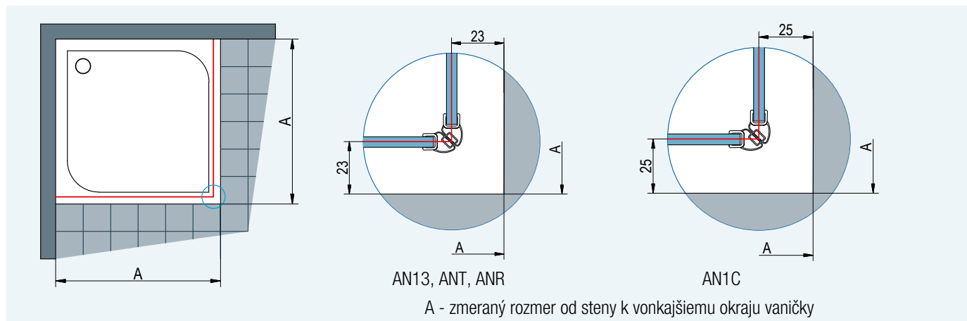
Obr. 1: Pri montáži na vaničku je odsadenie 23 mm (AN13, ANT, ANR), 25 mm (AN1C).
