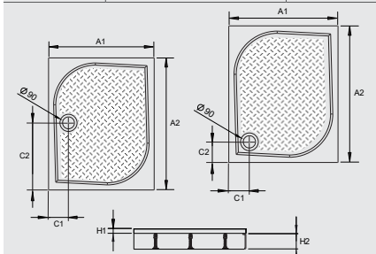
Sprchová vanička s nohami
