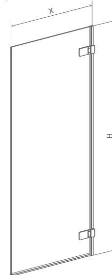
pravostranná vaňová zástena
