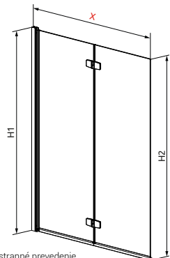
Lavostranné prevedenie vaňovej zásteny
