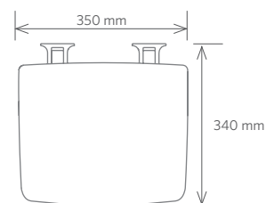
■ Sprchové sedátko Shower seat | Klappsitz Сиденье для душа 350 x 70 x 340 mm 203125074 2870,- Kč | 98,82 €
