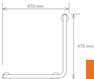
■ Madlo 90°, guma Grab bar 90°, rubber | Wannengriff 90°, Gummi Поручень 90°, резина 470 x 470 x 80 mm 104507731 pravé | right | recht | правый 104507721 levé | left | link | левый 1485,- Kč / 51,13 €
