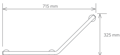
■ Madlo 135° Grab bar, 135° angled, | Wannengriff abgewinkelt 135° Поручень изогнутый 135° 715 x 325 x 80 mm 104507711 pravé | right | recht | правый 104507701 levé | left | link | левый 1480,- Kč / 50,96 €
