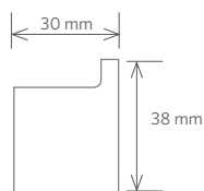
■ Věšáček Single robe hook | Kleiderhaken Крючок для одежды 17 x 38 x 30 mm 135006012 175,- Kč / 6,02 €
