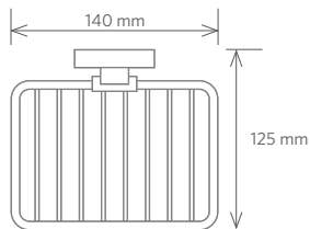
■ Mýdlenka Soap basket | Seifenhalter Мыльница 140 x 55 x 125 mm 104108160
