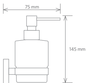
■ Dávkač tekutého mýdla, MINI Soap dispenser, MINI glass Seifenspender, MINI Дозатор жидкого мыла, MINI 75 x 145 x 100 mm, 200 ml 104109100
