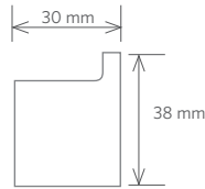
■ Věšáček Single robe hook | Kleiderhaken Крючок для одежды 17 x 38 x 30 mm 135006012
