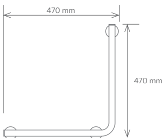
■ Madlo 90°, guma Grab bar 90°, rubber | Wannengriff 90°, Gummi Поручень 90°, резина 470 x 470 x 80 mm 104507731 pravé | right | recht | правый 104507721 levé | left | link | левый
