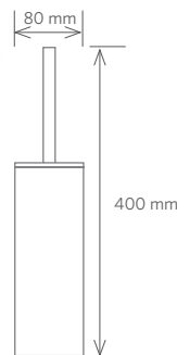
■ WC štětka na postavení nebo pověšení, nerez Toilet brush holder, free standing or hanging Bürstengarnitur Туалетная щетка с держателем (металл), напольный и настенный 80 x 400 x 80 mm 135913091
