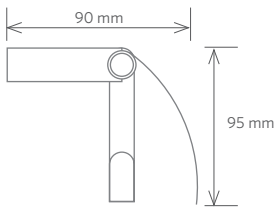
■ Držák toaletního papíru s krytem Paper holder with cover Papierrollenhalter mit Deckel Держатель туалетной бумаги с крышкой 130 x 95 x 90 mm 135012012
