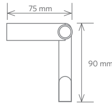
■ Držák toaletního papíru bez krytu Paper holder without cover Papierrollenhalter ohne Deckel Держатель туалетной бумаги без крышки 131 x 90 x 75 mm 135012222
