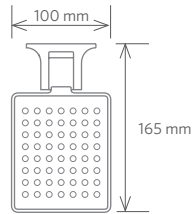
■ Nožní podpěra Footrest | Fußstütze Ножная опора 100 x 60 x 165 mm 203125084
