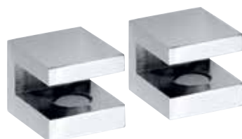
■ Držáky poliček pár Glass shelf holder - without glass, pair Halteung für Glasablagen, Paar Держатель полочки без стекла (пара) 20 x 20 x 25 mm, ≠ 8 mm 102202112
