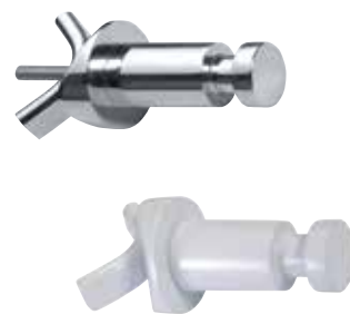
Háček na otopné těleso Radiator hook | Haken für den Handtuchhalter Крючок на радиатор 32 x 32 x 80 mm 104506122 lesk | polished | poliert | блеск 104506124 bílý | white | weiss | белый
