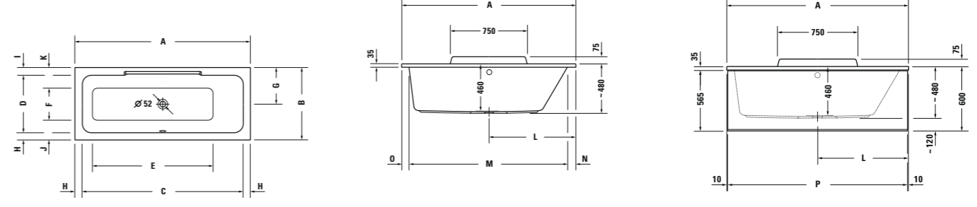
# 700293 00 00 0000, 1600 x 700 mm # 700295 00 00 0000, 1700 x 700 mm # 700297 00 00 0000, 1700 x 750 mm Einbauversion. Built-in. Da incasso. Version à encastrier. Inbouwversie. Versión empotrada *
