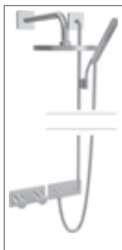
HANSALIVING Inštalčný balíček na konečnú montáž 10.1 batéria s termostatom, DN 15 (G1/2) hodiace sa k HANSAMATRIX 4487 0070 chróm 1.375,31 € vhodná pre HANSASIGNATUR, HANSALOFT, HANSADESIGNO, HANSALIGNA, HANSASTECLA, HANSARONDA, súprava s nástennou tyčou 1100 mm, s hlavovou sprchou HANSARAIN, DN 15
