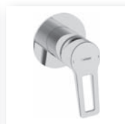
HANSATWIST Sada pro konečnou montáž pákové sprchové baterie, 4977 7005 chromovaná, třmenová páka 4977 7003 chromovaná, plná páka podomítkové těleso 5050 0100 objednejte samostatně
