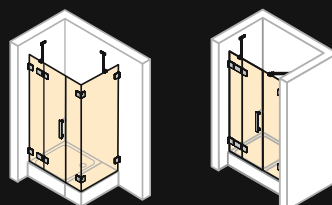
Křídlové dveře s pevným segmentem a protisegmentom
