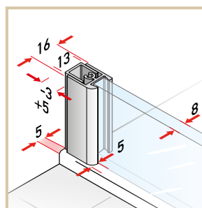
Pevný segment a boční panel
